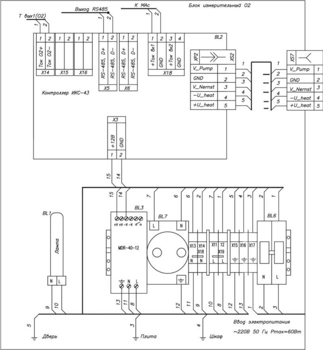
Рис. П 3 — Схема электрическая соединений блока O2
