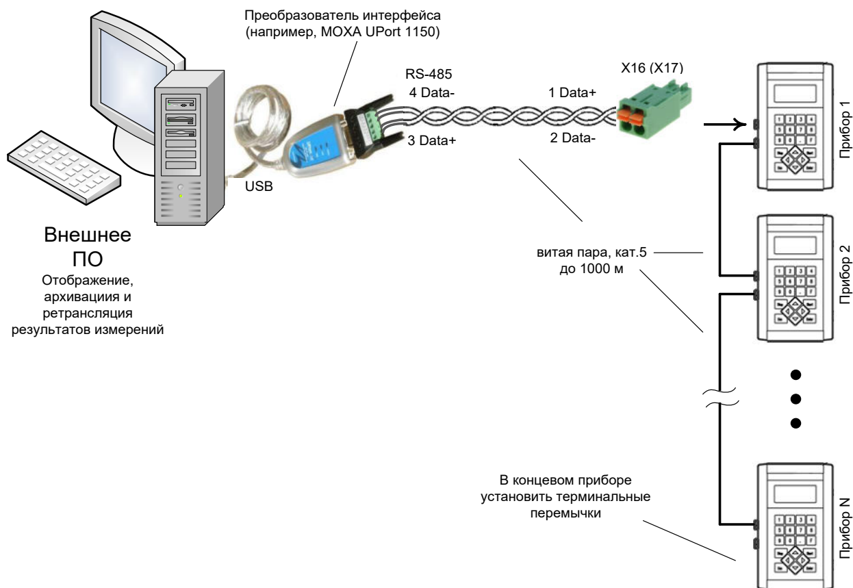
Схема кабеля связи ПЭВМ – ИКТС-11
